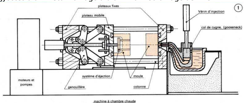
machine à chambre chaude
