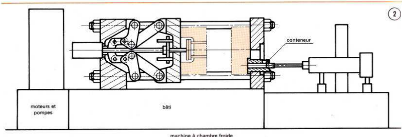
Schémas des machines à chambre chaudes et à chambre froide
